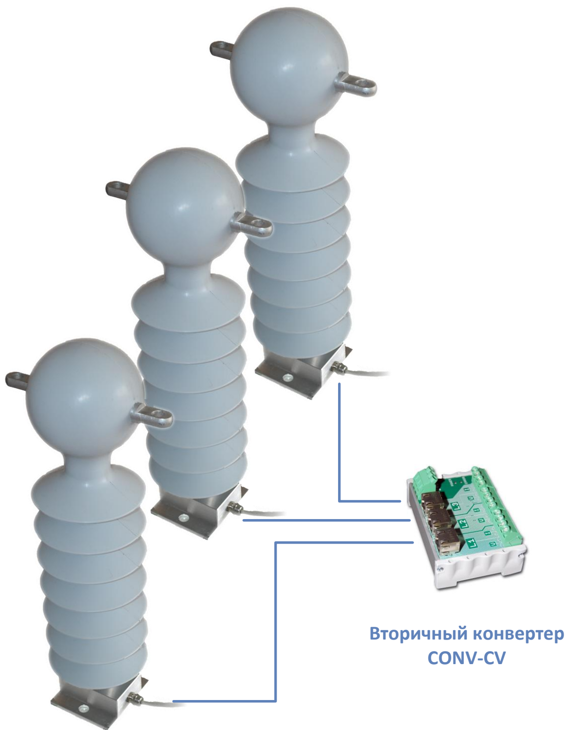
Первичный преобразователь CVS-O-35 (3 Фазы)
